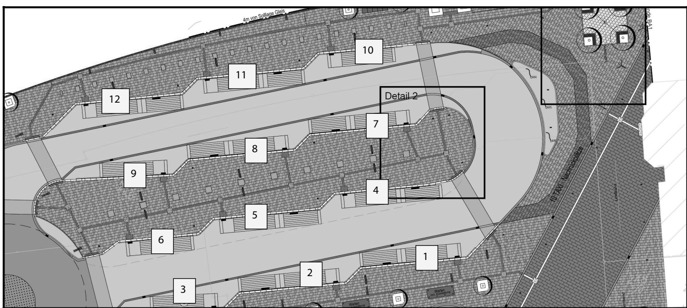
Haltepunktbelegung am neuen Bahnhof/ZOB Wetzlar
